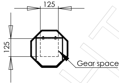
SECTION A-A SCALE 1 : 15
